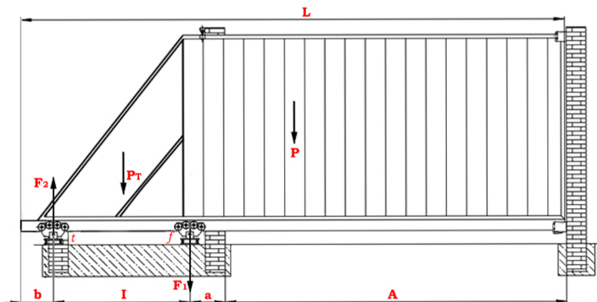
Рис.1 Схема сил, действующих на элементы конструкции ворот, кроме ветровых.
